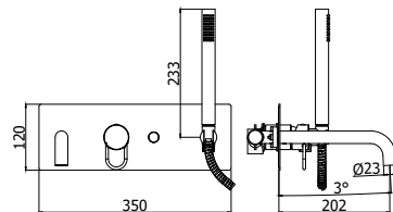
JK 001CR Miscelatore incasso vasca/doccia completo di deviatore, bocca e set doccia Concealed bath/shower mixer with diverter, spout and shower kit
