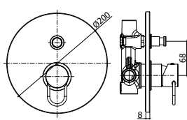
JK 015CR Miscelatore incasso doccia (2 uscite) con deviatore a pulsante Concealed shower mixer (2 outlets) with push diverter
