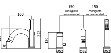
JK 041L-040LCR Miscelatore bordo vasca con doccia estraibile, con/senza bocca erogazione Deck mounted bath mixer with pull out hand-shower, with/without spout
