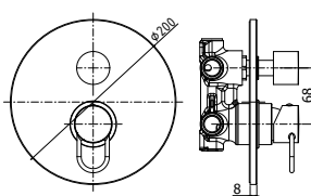
JK 018CR Miscelatore incasso doccia (2 uscite) con cartuccia deviatore Concealed shower mixer (2 outlets) with diverter cartridge
