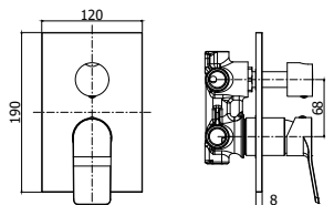
TI 019CR Miscelatore incasso doccia (3 uscite) con cartuccia deviatore Concealed shower mixer (3 outlets) with diverter cartridge
