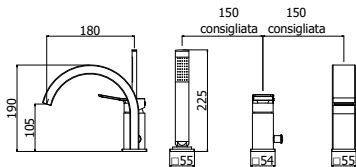
TI 040-041CR Batteria miscelatore bordo vasca con doc- cia estraibile, con/ senza bocca erogazione Deck mounted bath mixer with pull out hand-shower, with/ without spout
