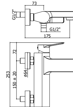
TI 022-023CR Miscelatore vasca doccia con/ senza set doccia Bath/shower mixer with/ without shower set
