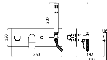
TI 001CR Miscelatore vasca incasso completo di deviatore, bocca e set doccia Concealed bath/shower mixer with diverter, spout and shower kit
