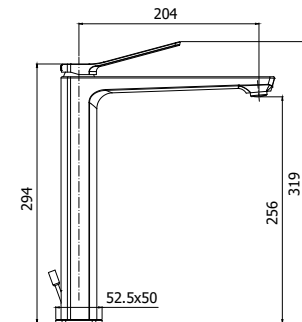
TI 081-085CR Miscelatore lavabo prolungato con/ senza scarico Tall wash basin mixer with/ without pop up waste
