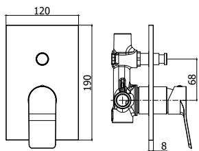
TI 015CR Miscelatore incasso doccia (2 uscite) con deviatore a pulsante Concealed shower mixer (2 outlets) with push diverter
